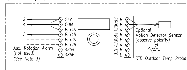
Optional Stop/Jog Controller:
